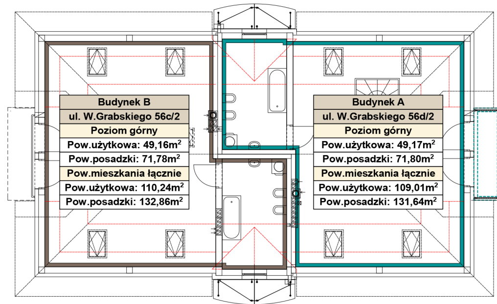
RZUT PODDASZA
