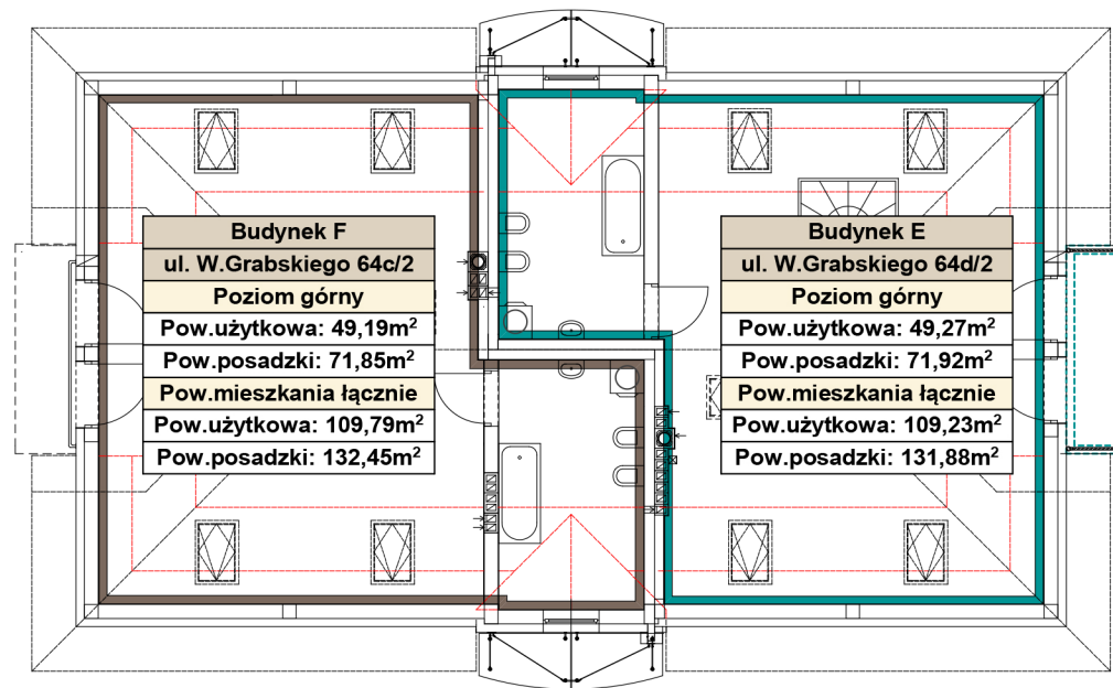
RZUT PODDASZA
